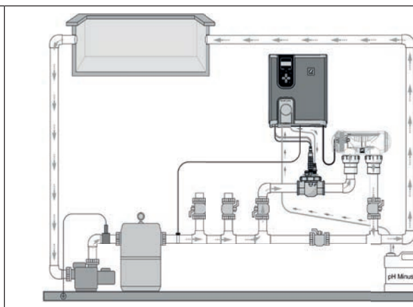
Instalación del aparato + módulo opcional
